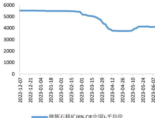
图表 5 锂辉石精矿现货价格（单位：元/吨）
