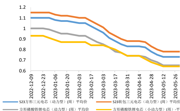
图表 15 各类电芯价格走势（单位：元/吨）
