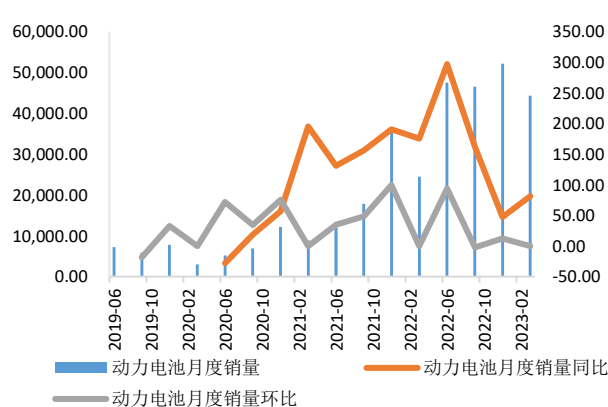
图表 27 锂电池月度销量、同比、环比（单位：MWh、%、%）
