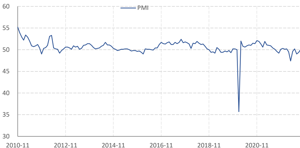
图表 4: PMI
