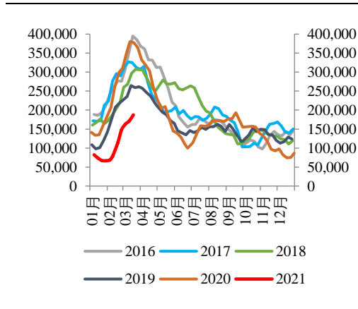
图9: 上期所库存 (单位: 吨)
