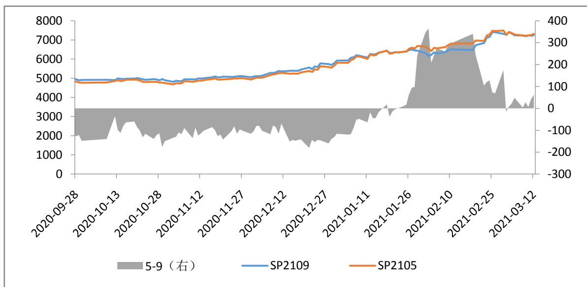
图：SP2105 与 SP2109 收盘价对比图
