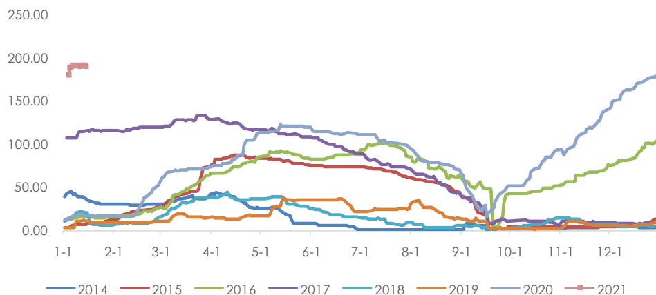
图 4：仓单（万吨）
