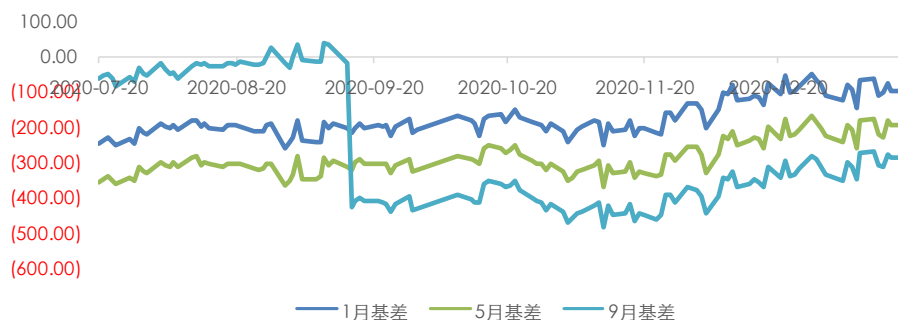
图 1：PTA 基差
