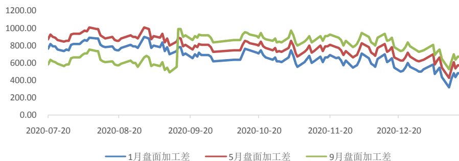
图 3：盘面加工差
