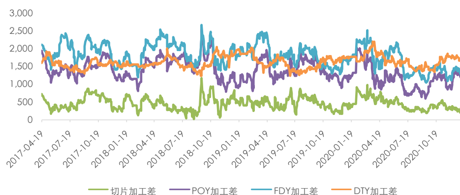
图 13: POY、FDY、DTY 加工差
