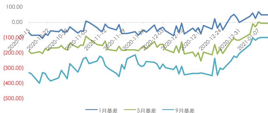
图 7：MEG 基差
