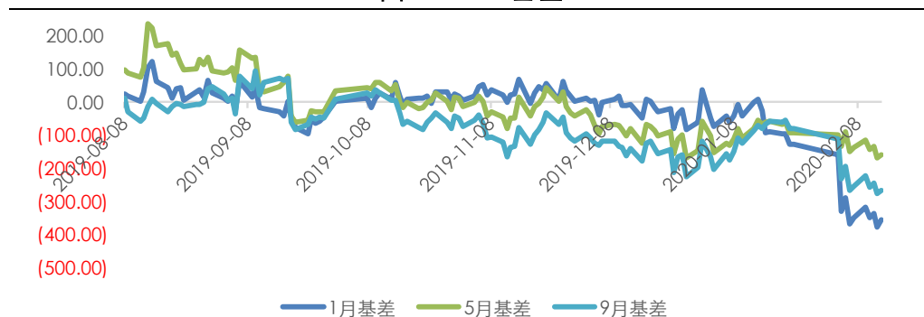
图 1: PTA 基差
