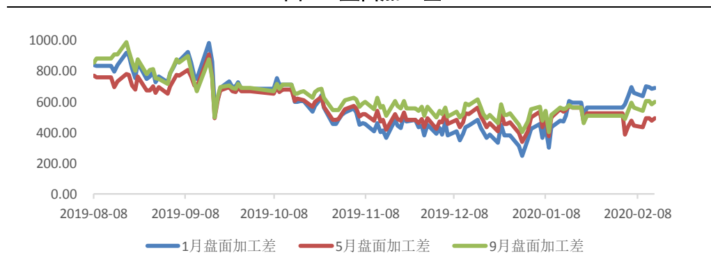
图 3: 盘面加工差
