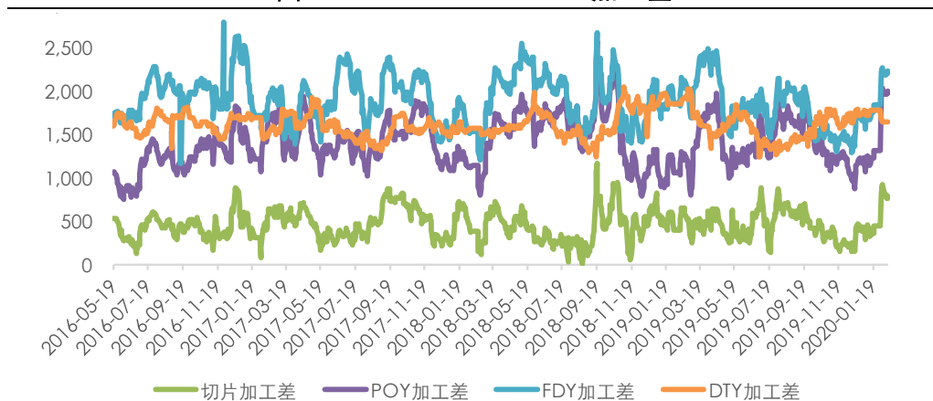
图 13: POY、FDY、DTY 加工差
