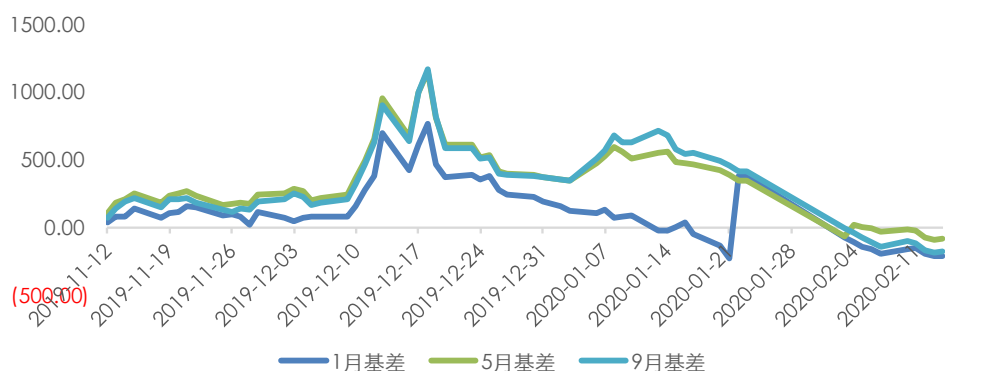
图 7：MEG 基差
