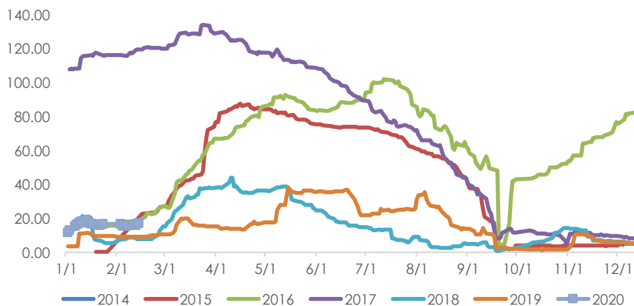
图 4：仓单（万吨）
