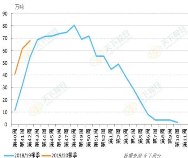
图 7：甜菜压榨量
