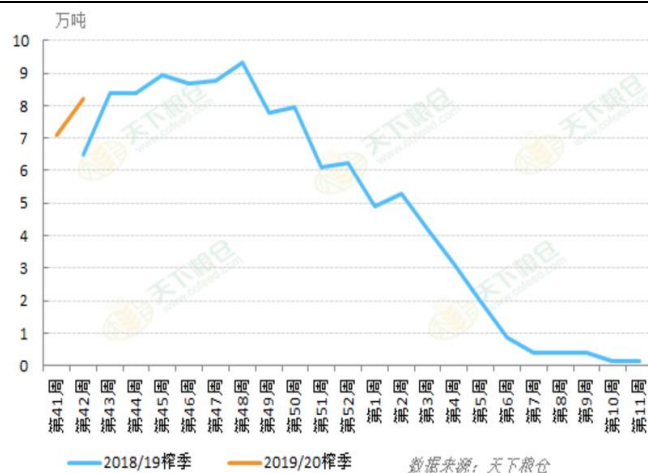
图 8：甜菜糖产量
