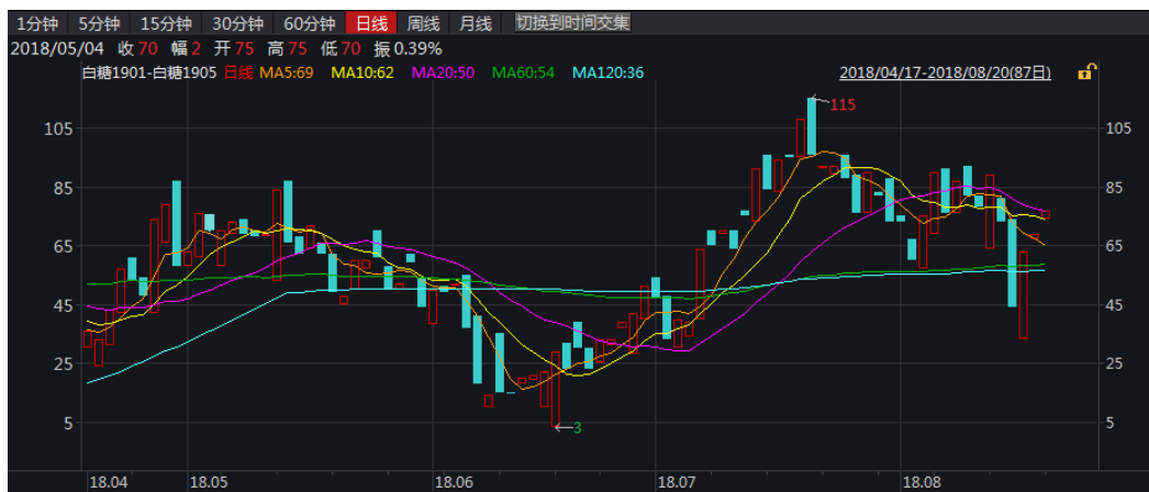
图 1: 郑糖 1-5 价差
