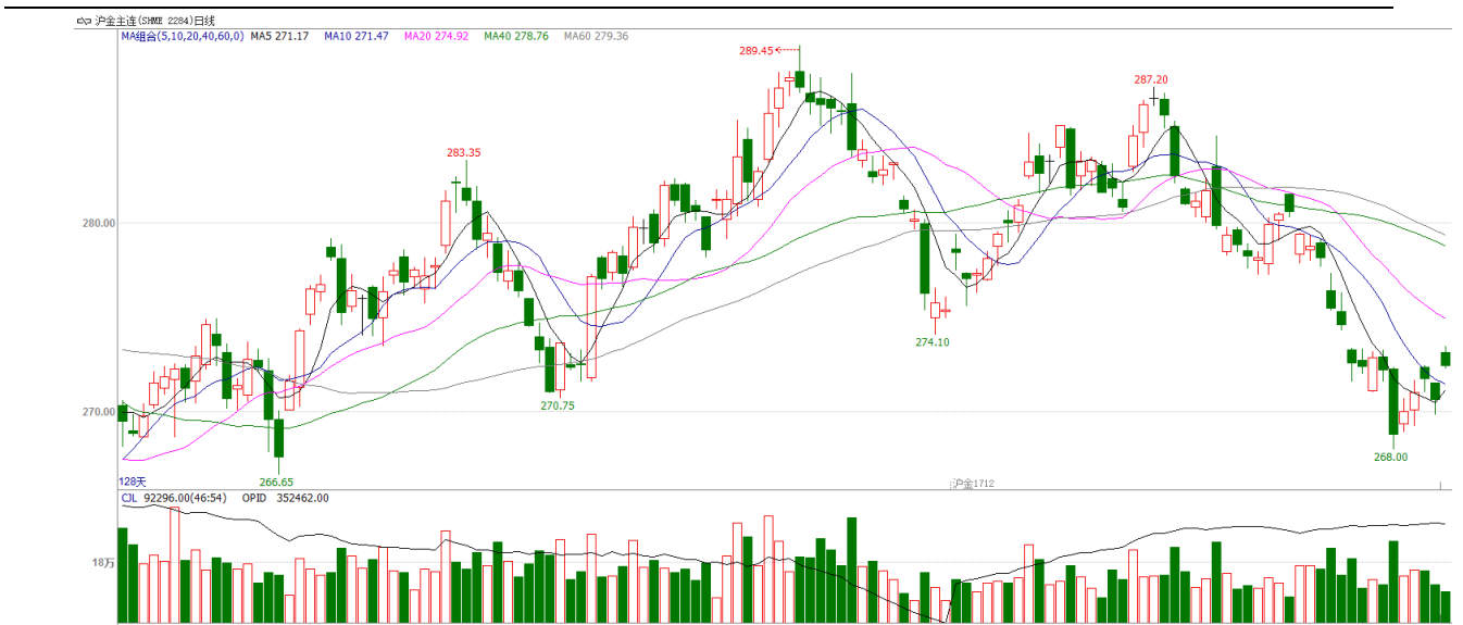
图 2: 沪金 1712 合约
