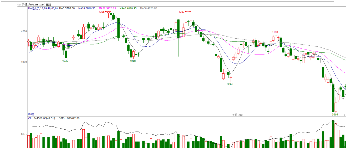
图 4：沪银 1712 合约
