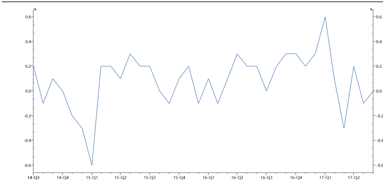
图 10：美国 6 月 CPI
